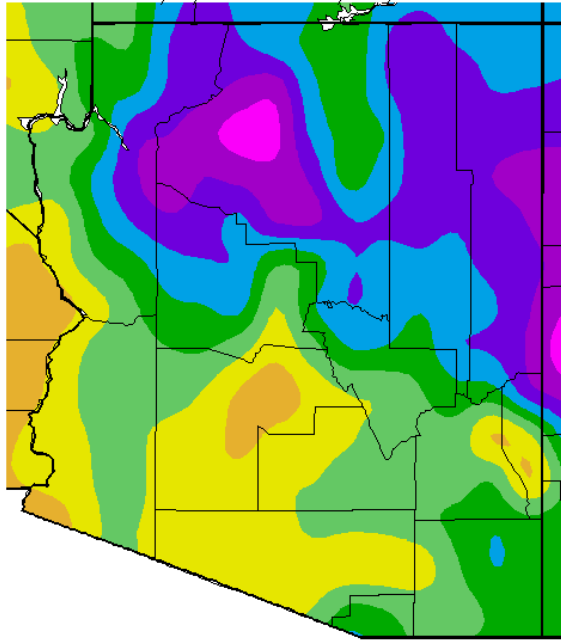
Av. Min. Temperature (deg. F) 3/1/2009 – 3/31/2009
